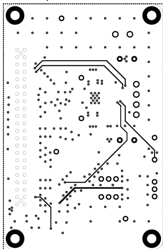
3 - Inner Layer 2
